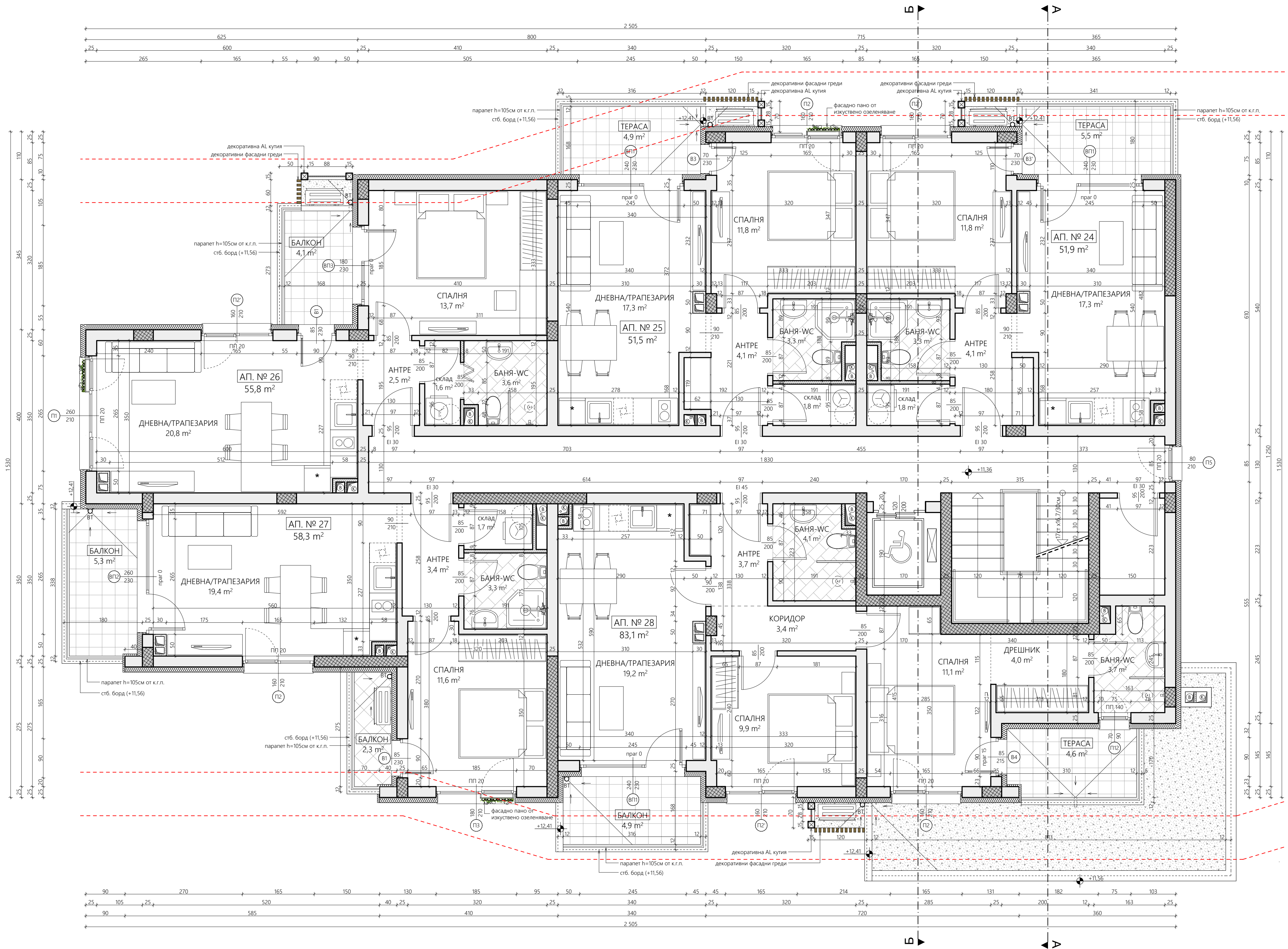
Разпределение на кота +11,36 (ПЕТИ ЕТАЖ) М 1:50
