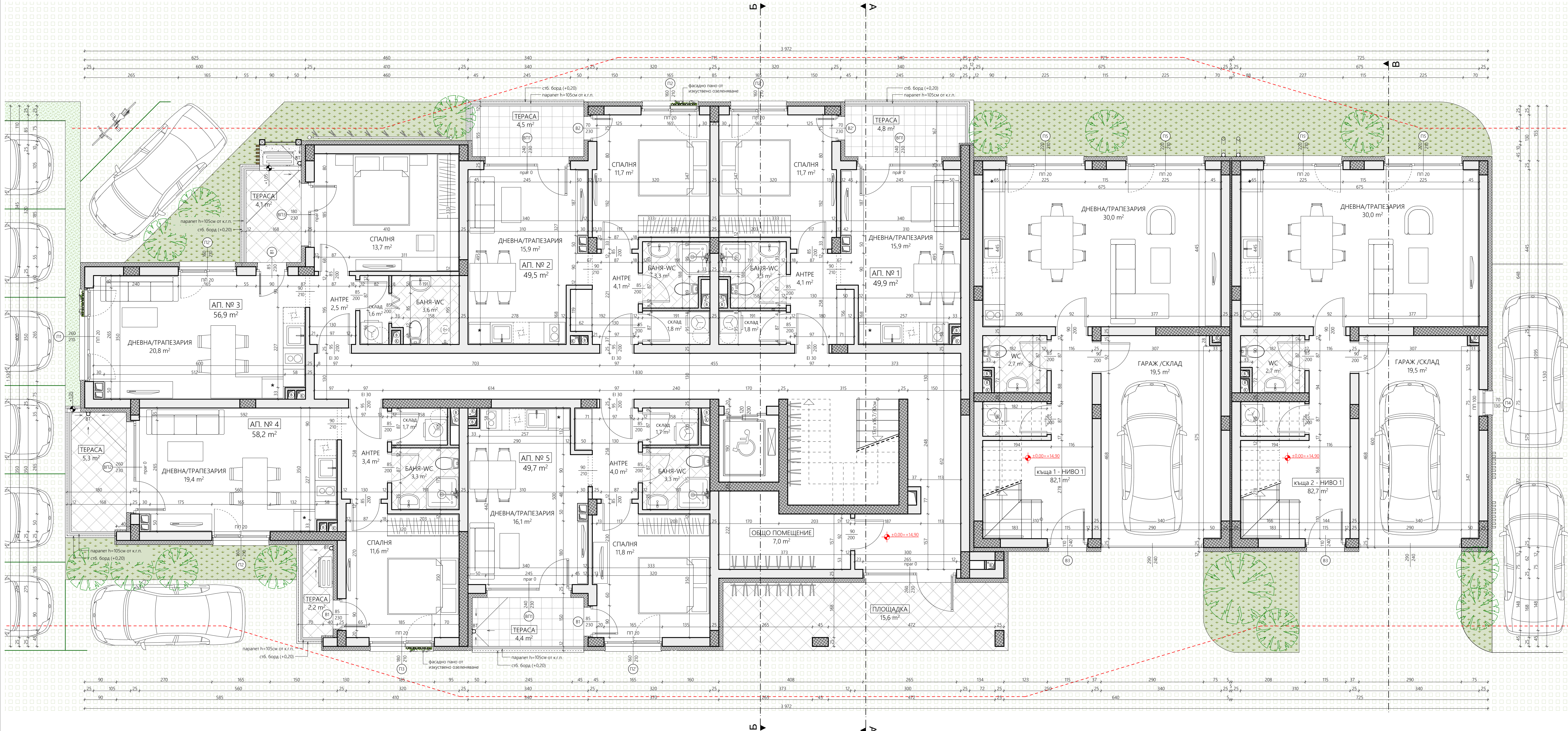
Разпределение на кота ±0,00 (ПЪРВИ ЕТАЖ) М 1:50
